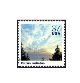
Cirrus radiatus
